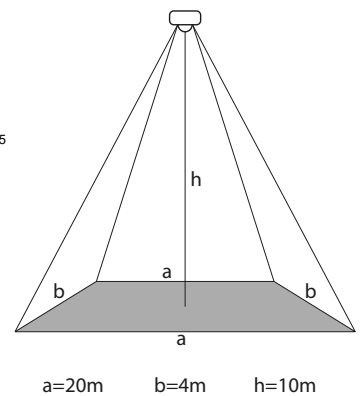
Pole detekcji czujnika SES08WH
