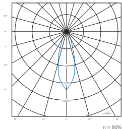
► OGR50 JDR 35W
