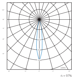
► OGR50 LED HP 3W
