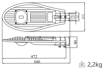
► KUL1-050BL-6K
