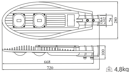
► KUL1-100BL-6K
