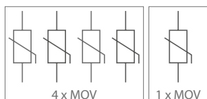
ogranicznik warystorowy
