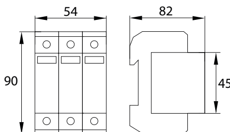
► SPD-MOV-DC-3P-T1T2
