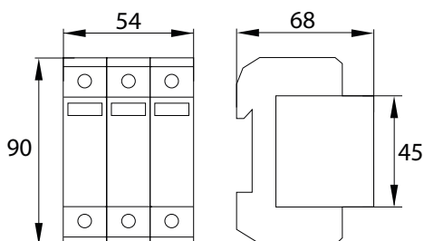
► SPD-MOV-DC-3P-T2
