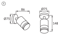
① TARAS SPT GU10 INOX
