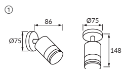
① TARAS SPT GU10 INOX
