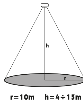
Pole detekcji czujnika SES68WH
