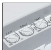
SES73WH - regulacja płynna: TIME, SENS, LUX
