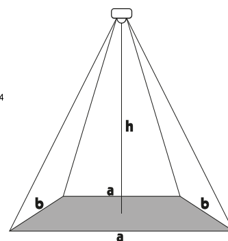
Pole detekcji czujnika SES08WH
